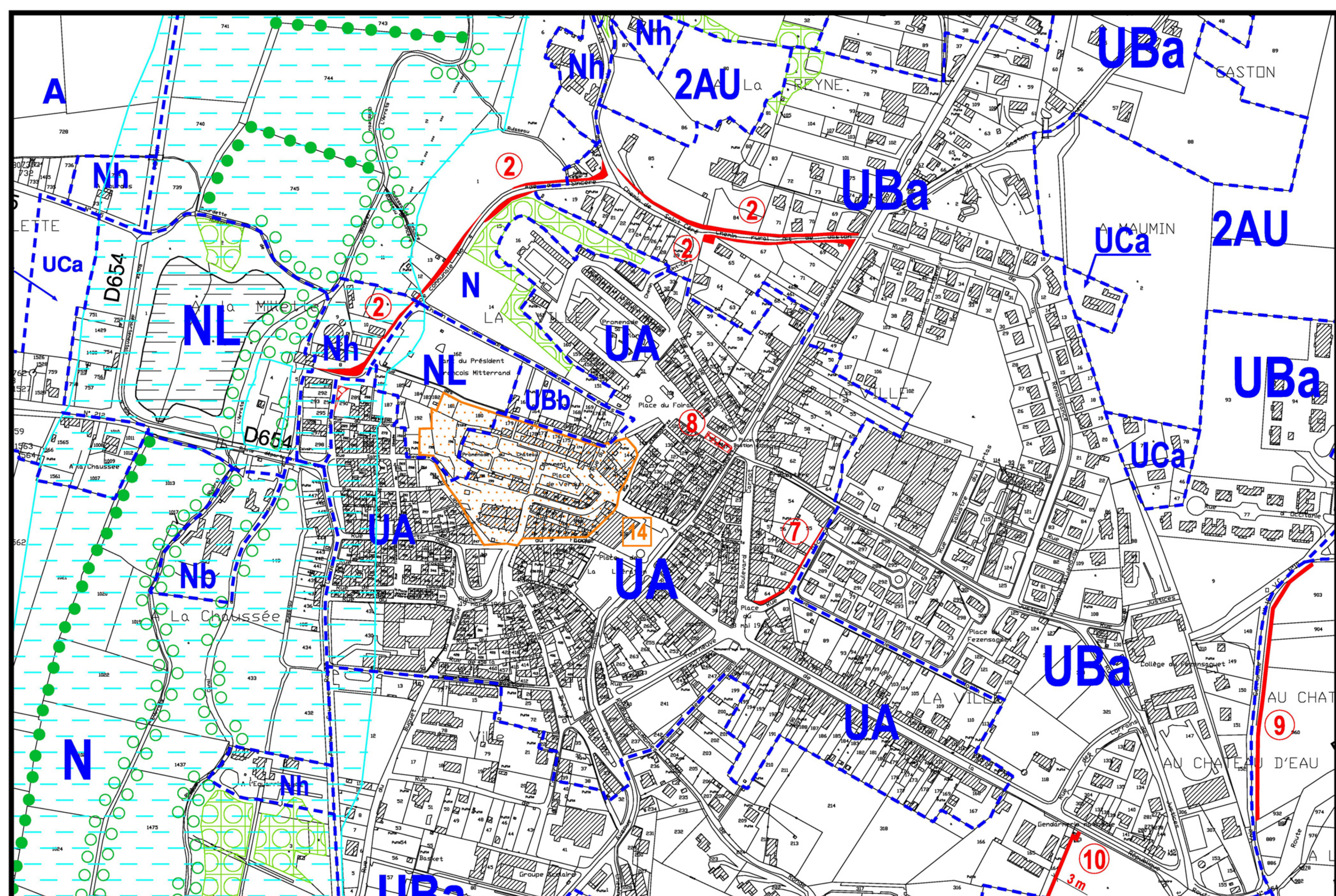
Echelle 1/2500
